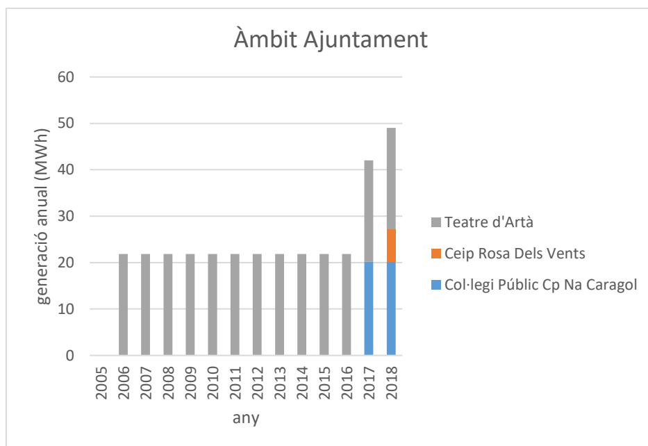
Gràfica 25: Producció fotovoltaica en l'àmbit Ajuntament. Font: Elaboració pròpia a partir de dades facilitades per l'Ajuntament.
