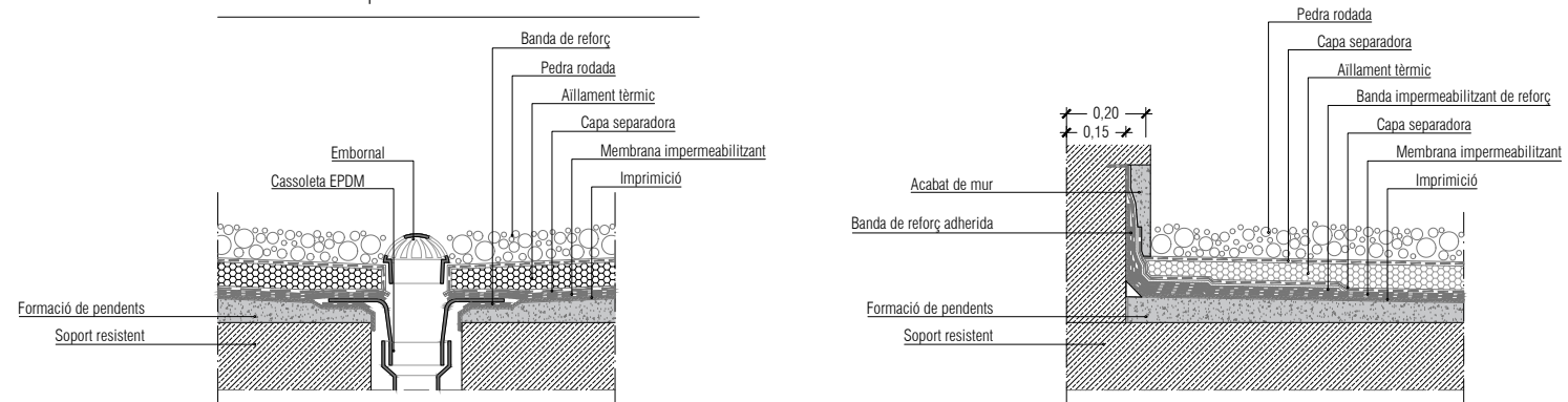
DETALLS - Coberta plana invertida no transitable
