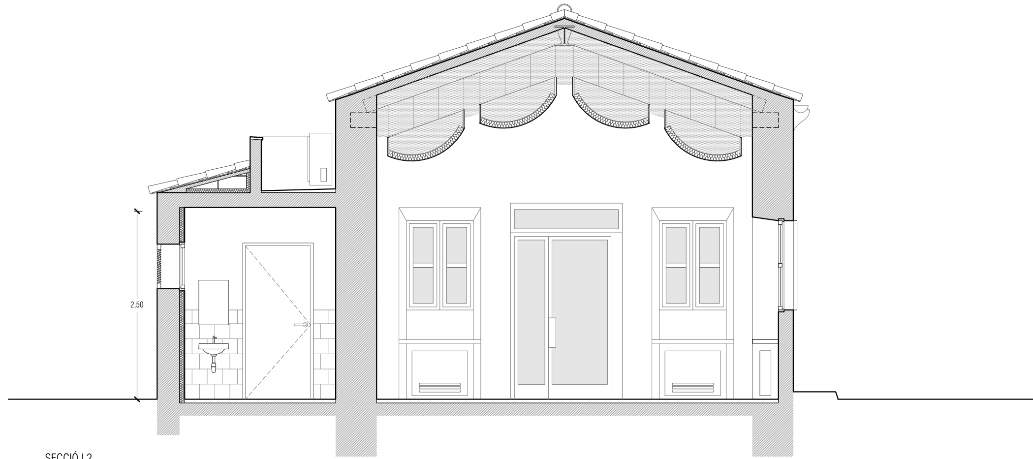
SECCIÓ L2
