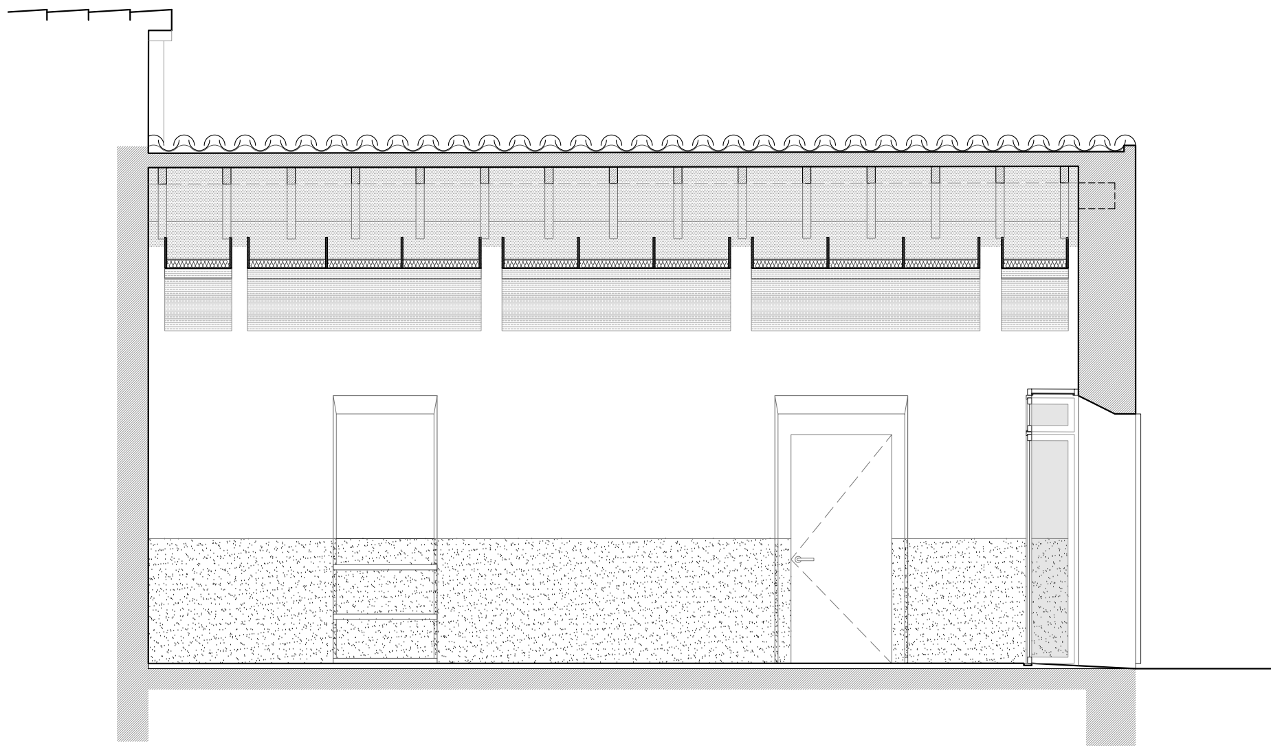
SECCIÓ T1
